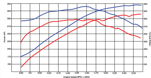
Dyno Chart
