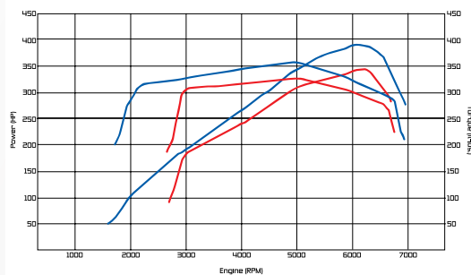
Dyno Chart
