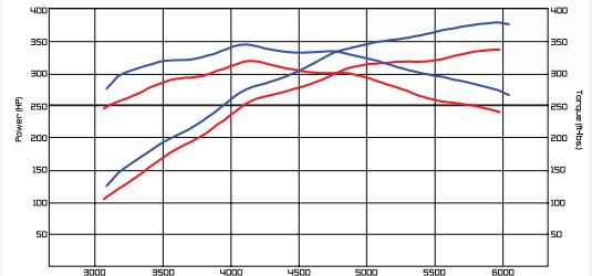
Dyno Chart
